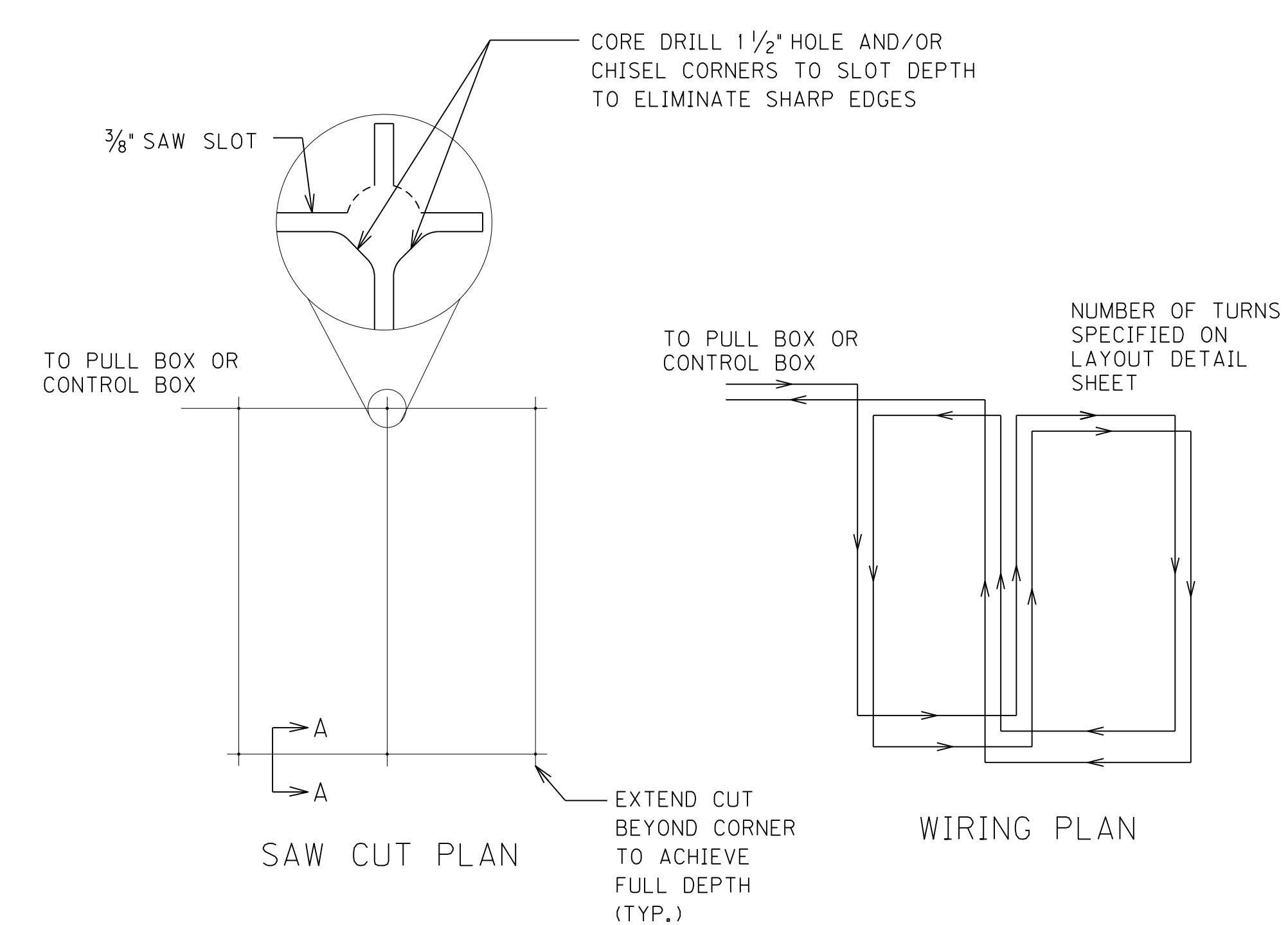
6'x30' QUADRAPOLE LOOP
